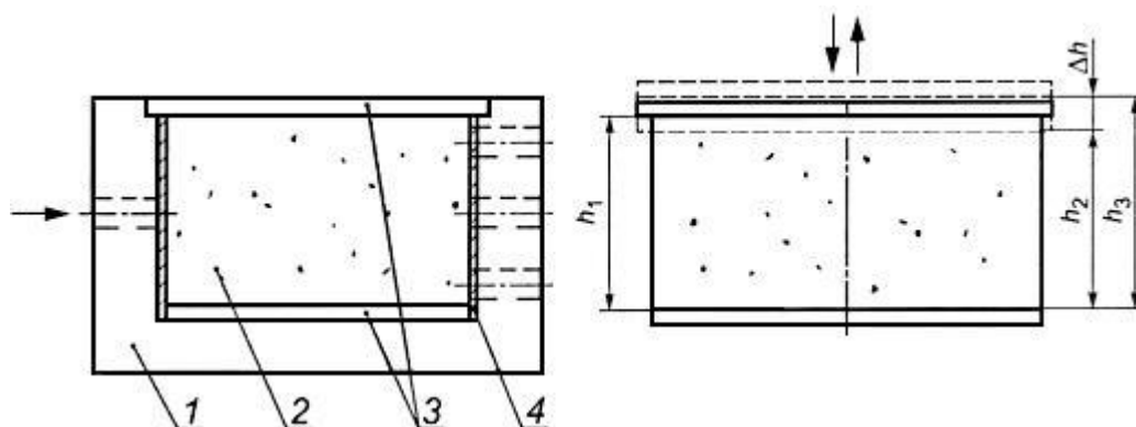
Рисунок 3 - Схема устройства для подготовки образца и испытания пенного утеплителя на деформационную устойчивость
