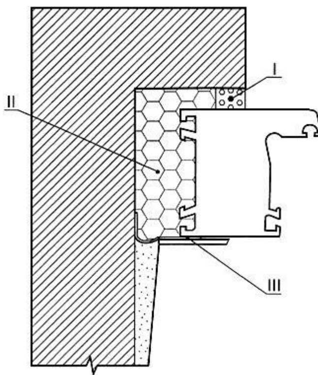
Рисунок 1 - Принципиальная схема монтажного шва
