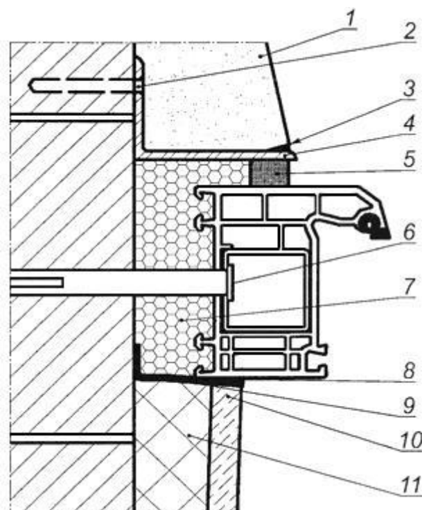
Рисунок А.2 - Узел бокового примыкания оконного блока к проему без четверти в стене из кирпича и с отделкой внутреннего откоса облицовочной панелью
