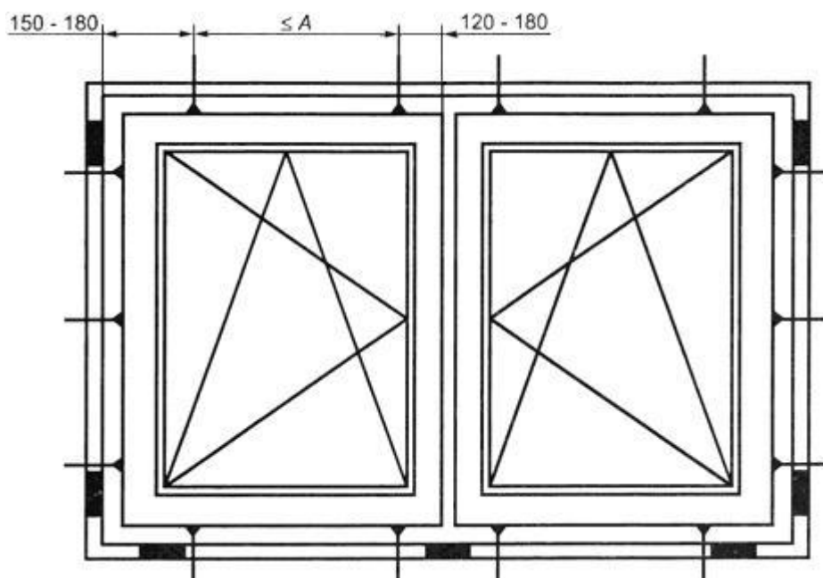
Рисунок Б.1 - Пример расположения точек крепления коробки и опорных (несущих) колодок и крепежных деталей
