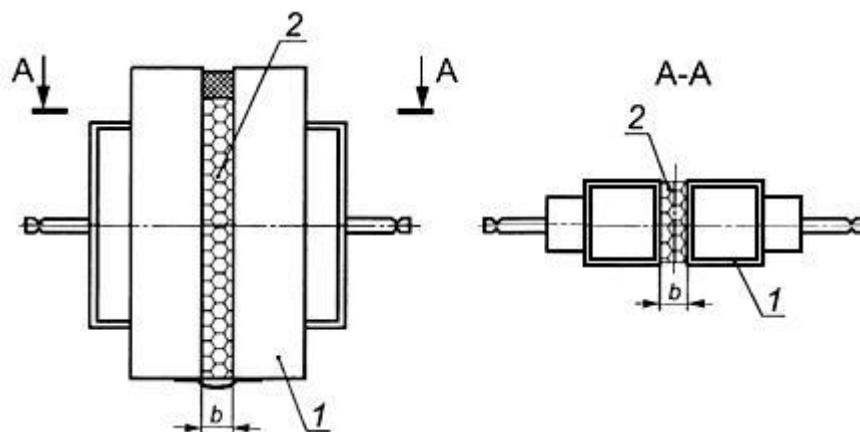
Рисунок 2 - Схема приспособления для испытания прямых монтажных швов на деформационную устойчивость
