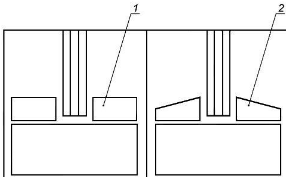
1 - прямоугольный штапик; 2 - скошенный/наклонный штапик
