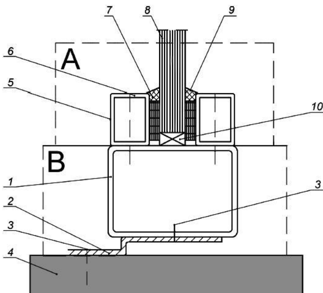
Рисунок 1 - Система остекления и система рамы
